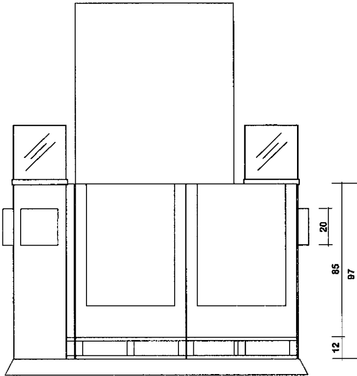
PROSPETTO FRONTALE
