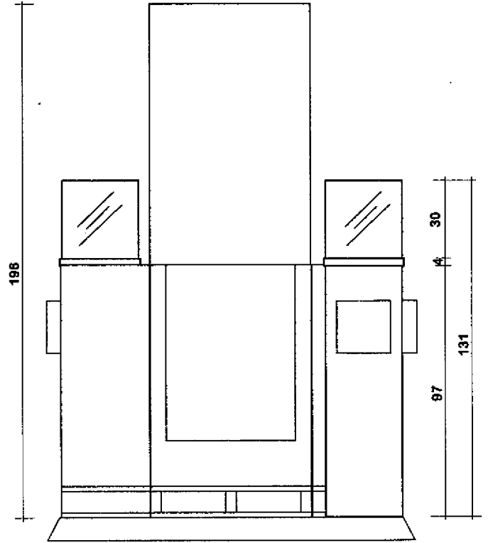
PROSPETTO LATERALE
