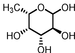
L-fucose
