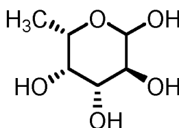
L-fucose
