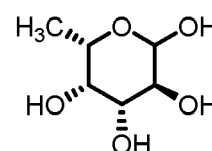
L-fucose;
