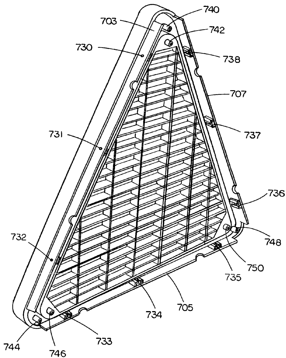
FIG. 15B
