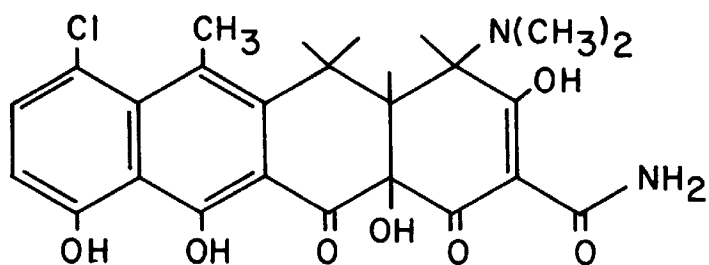
Anhydrochlortetracycline
