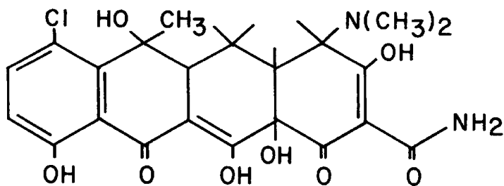
Chlortetracycline
