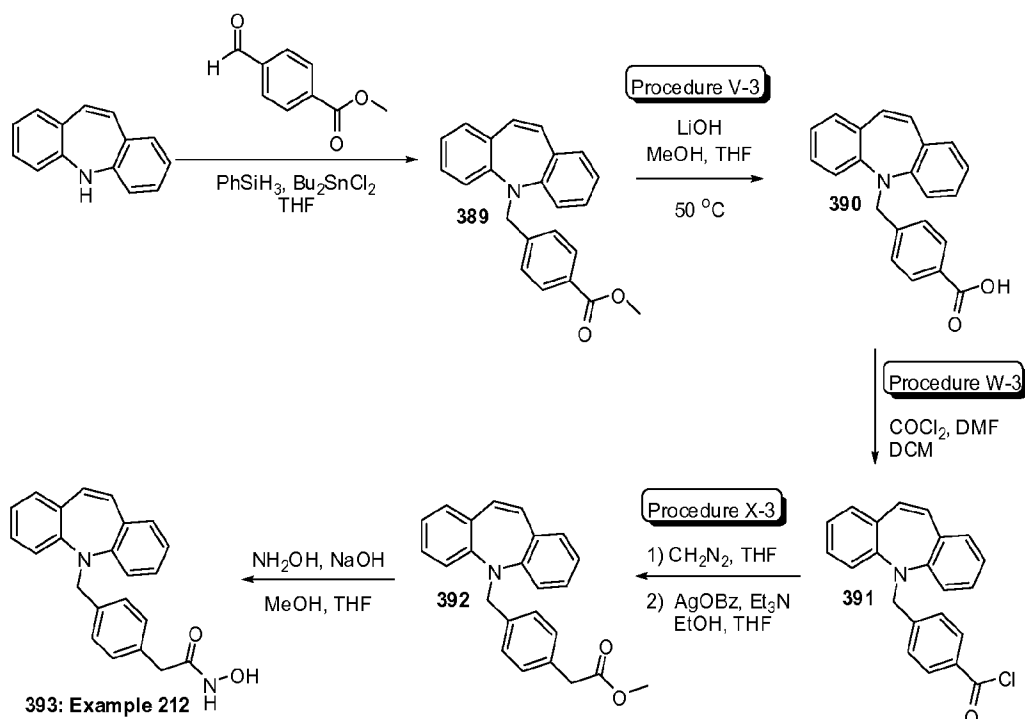
Example 212
