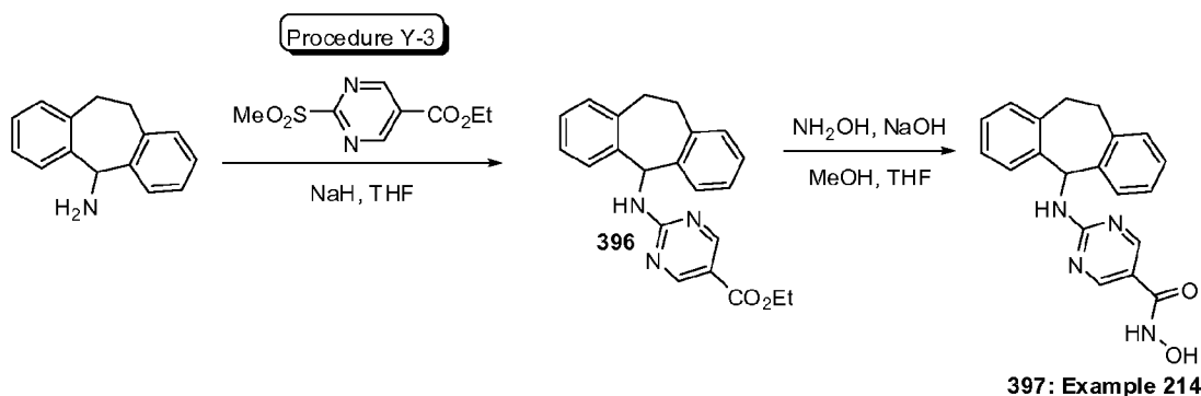
Example 214
