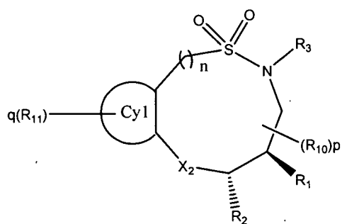
10 Formula IC
