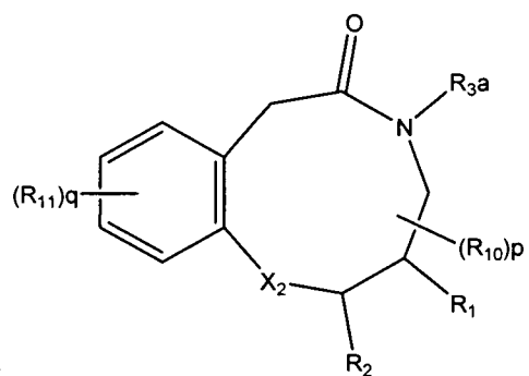
10 Formula VA
