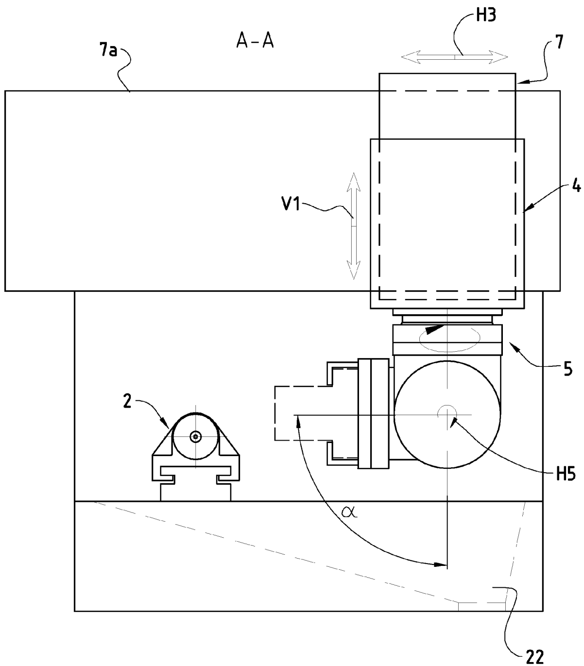
FIG. 7a
