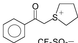
\text{CF}_3\text{SO}_3^- ( z 30)
