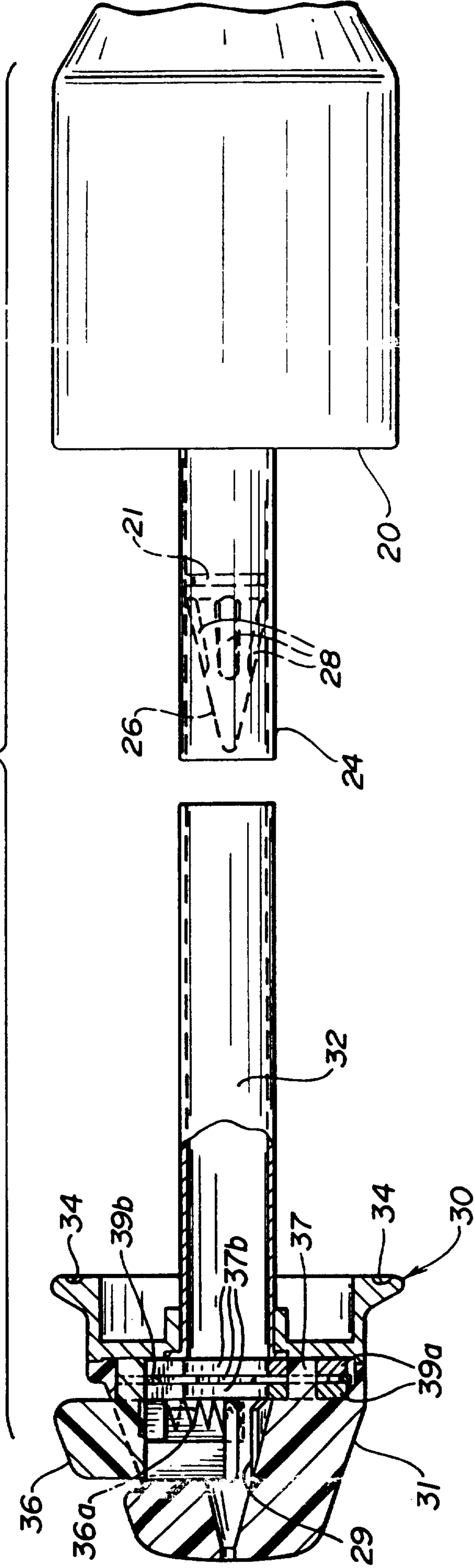
FIG-8
