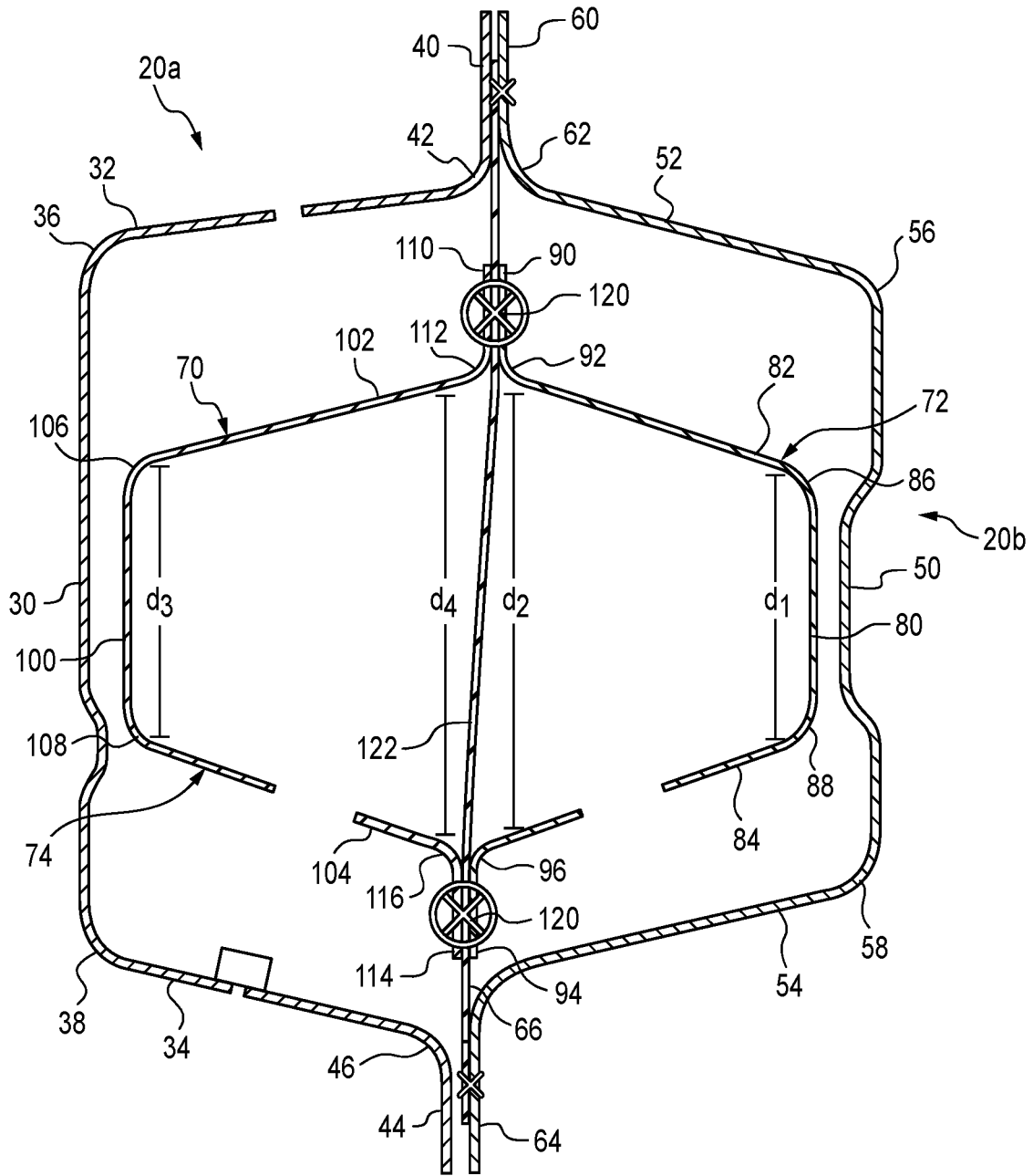
SECTION B-B FIG. 6
