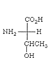
蘇胺酸
