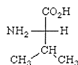
纈胺酸
