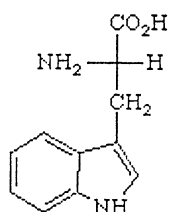
色胺酸
