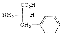
苯基丙胺酸
