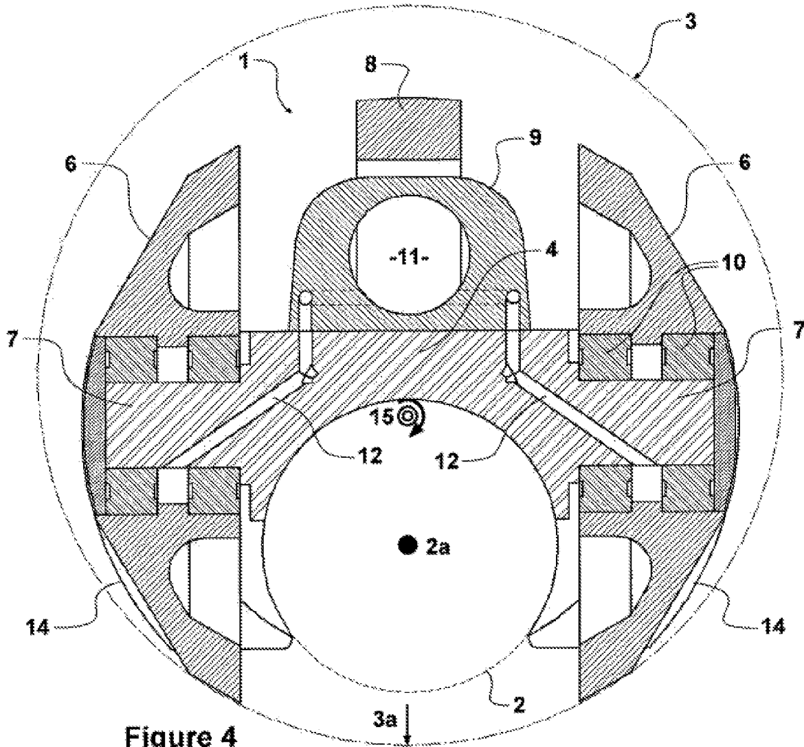
Section A-A
