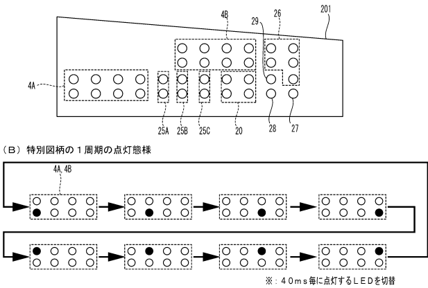
【図10-18】 (A) 特図ユニット
