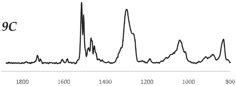
244 spectra, SNR 269
