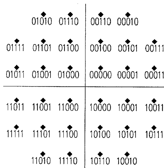
FIG. 12d 5 BITS PER BAUD
