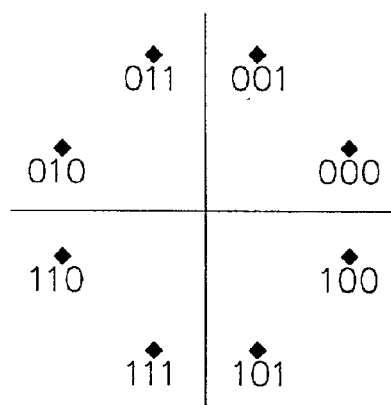
FIG. 12b 3 BITS PER BAUD
