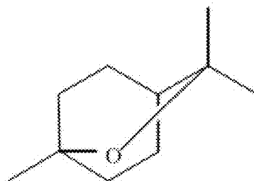
1,8-cineole
