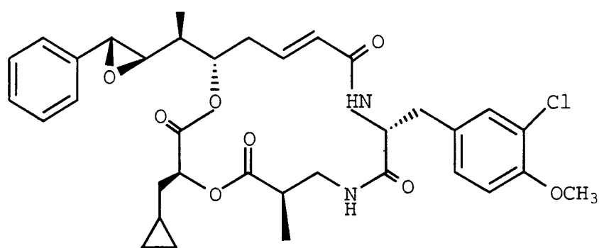
D-1
