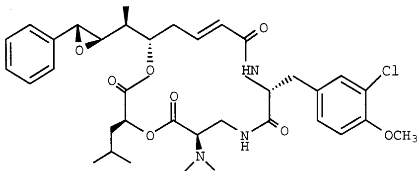
C-4
