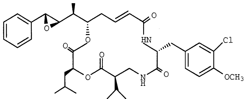
C-2
