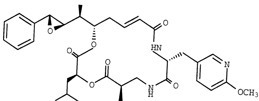
B-5
