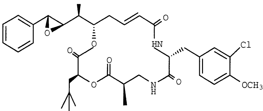
D-2
