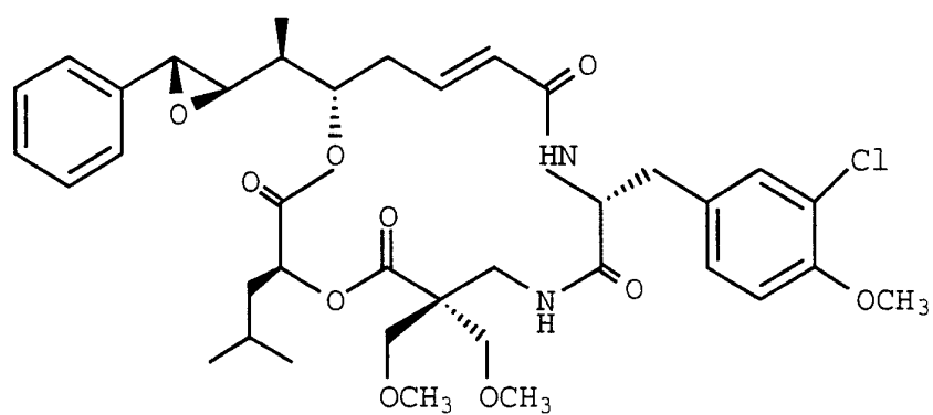
C-7
