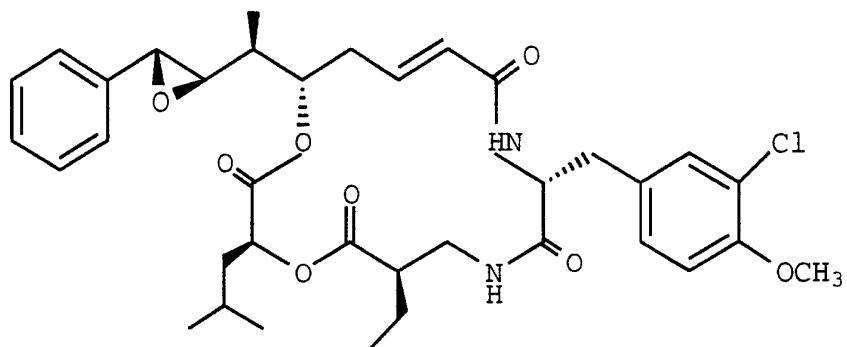
C-1
