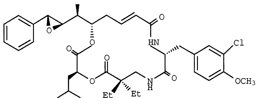
C-6
