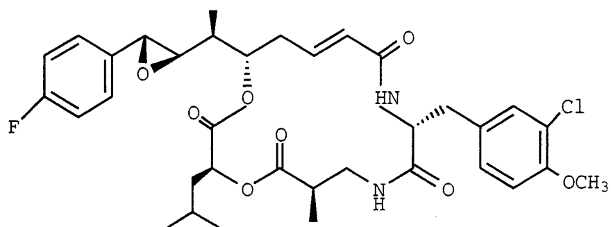
CRYPTOPHYCIN-189
