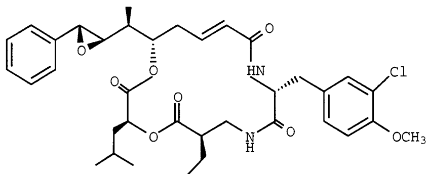
C-1
