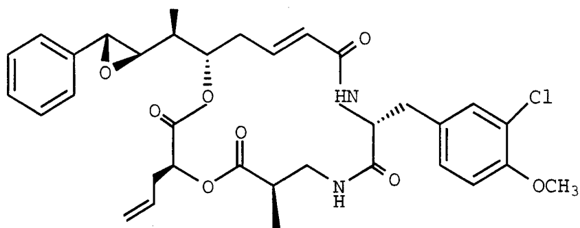
D-3
