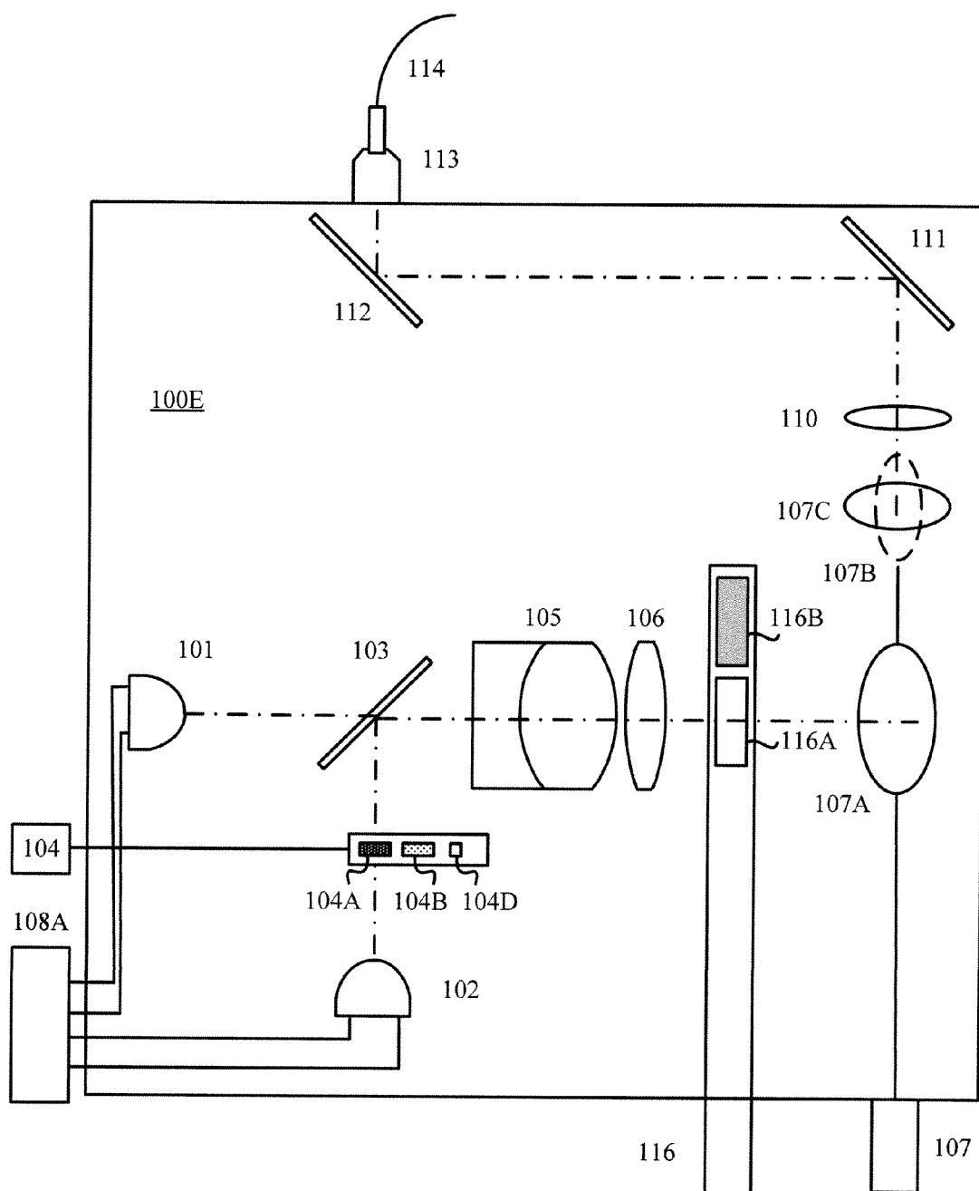
FIG. 1E
