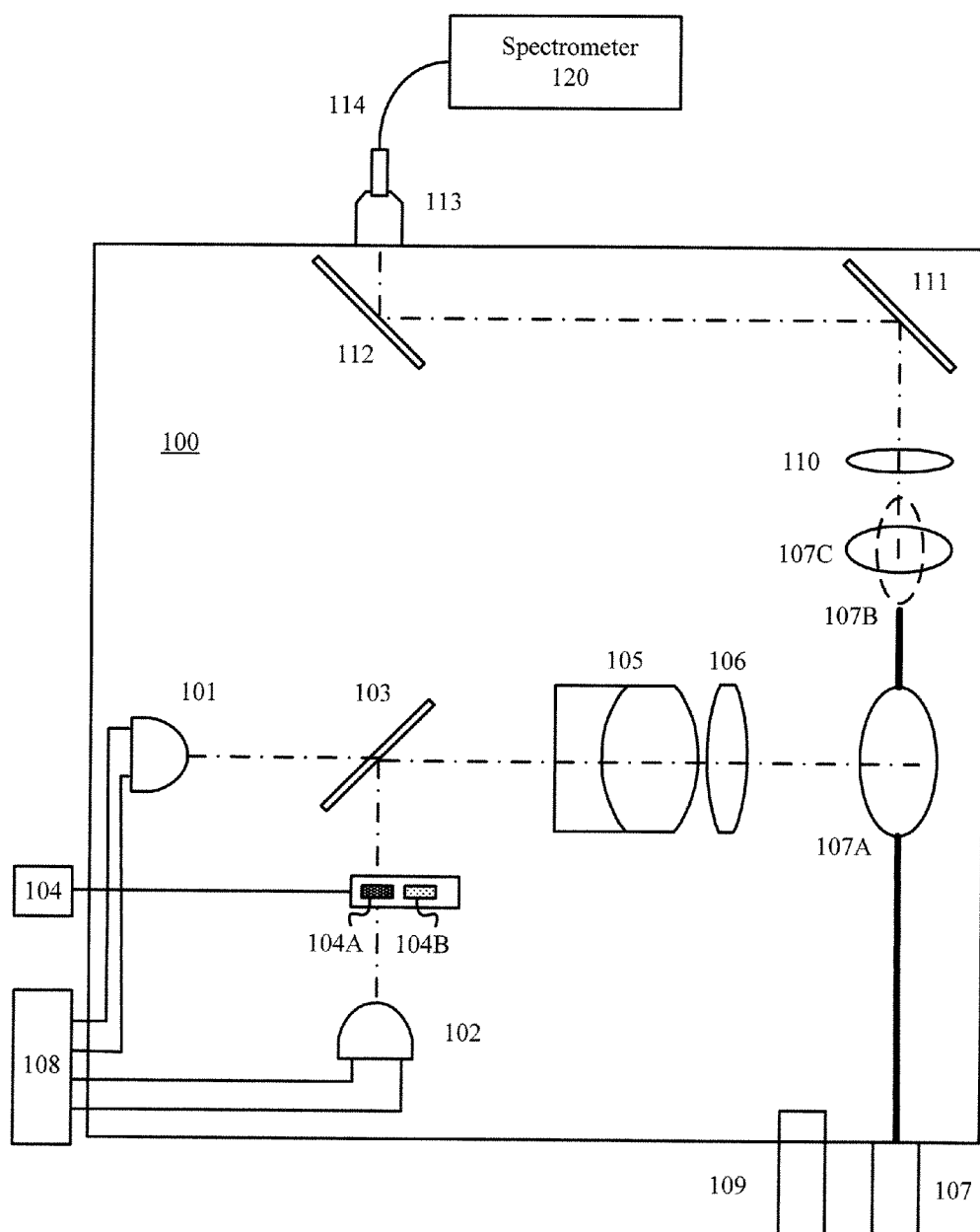
FIG. 1A
