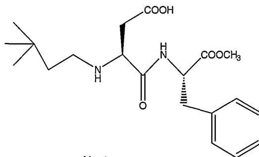
Neotame
