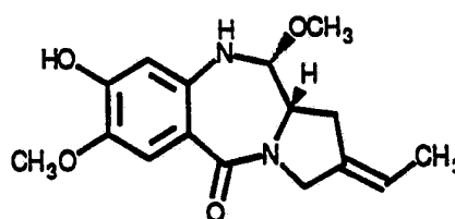
TOMAYMYCIN
