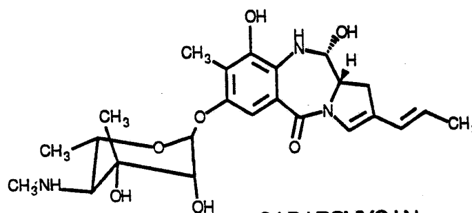
SIBIROMYCIN
