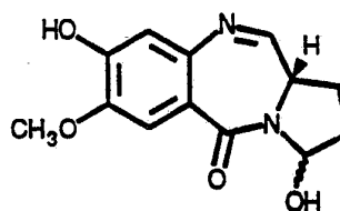
NEOTHRAMYCIN
