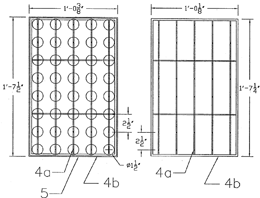
FIG. 8A: TOP VIEW
