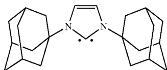
1,3-Bis(1-adamantyl)imidazol-2-yliden (Im-4)
