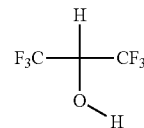
HFIP
