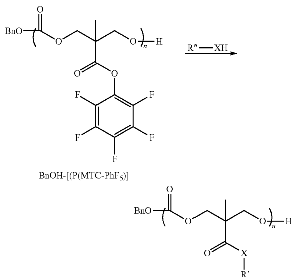
Scheme D.
