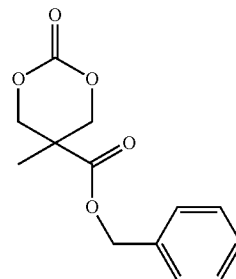
(MTCOBn)
