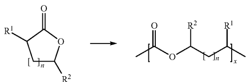
Scheme A.
