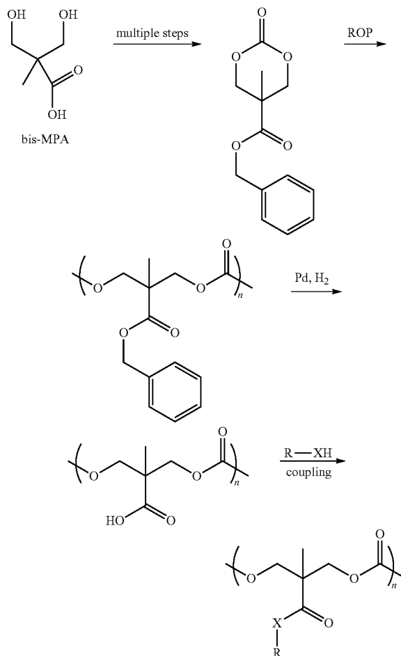
Scheme B.
