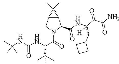
Boceprevir
