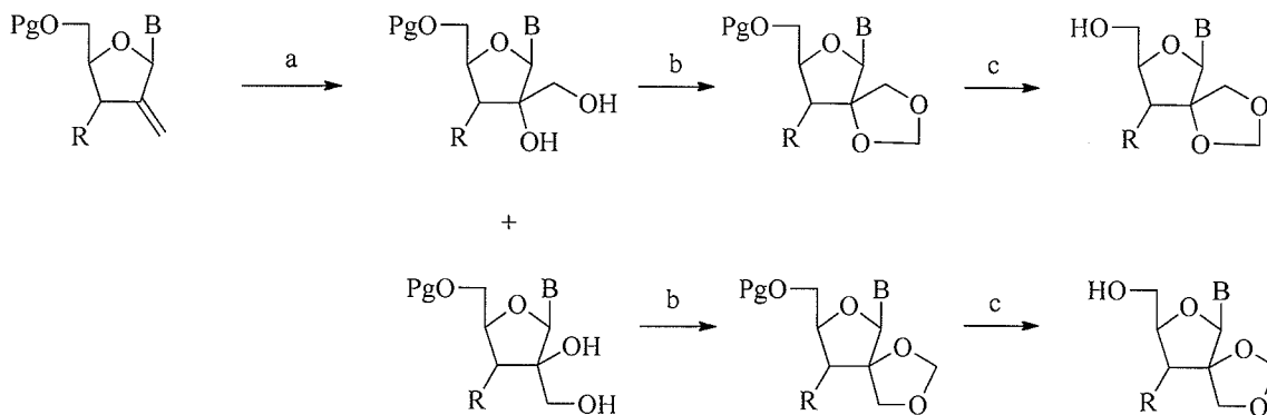
Scheme 3: Reagents: a) \text{OsO}_4/\text{NMO} ; b) \text{HCHO}/\text{acid} ; c) deprotection
