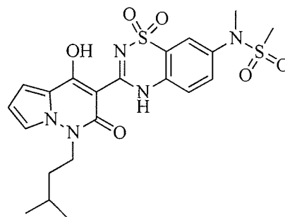
ANA-598
