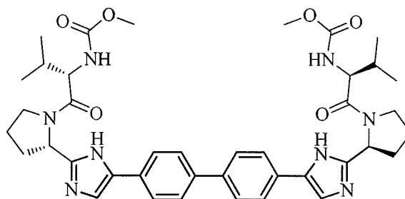
BMS-790052
