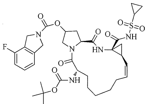
ITMN-191
