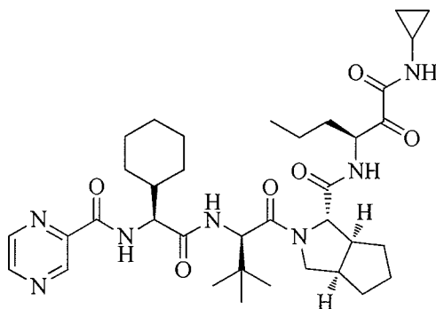
Telaprevir (VX-950)
