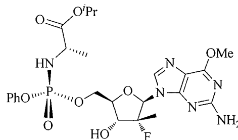
PSI-353661
