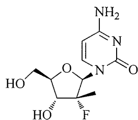
PSI-6130
