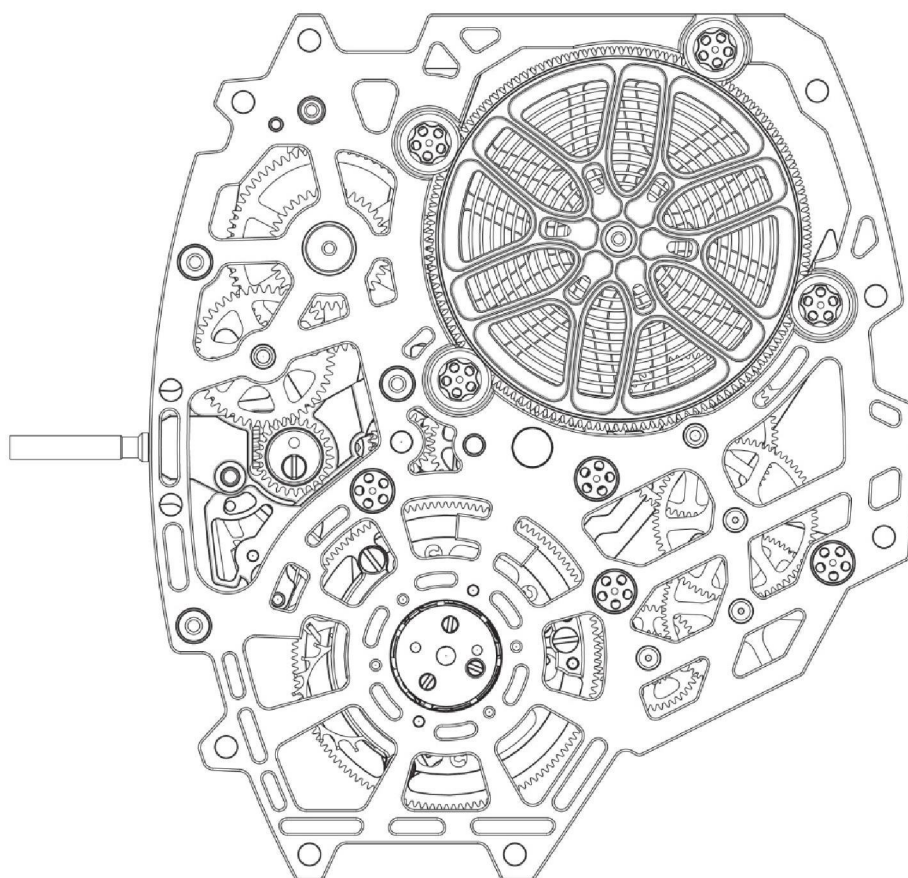
【後視圖】
