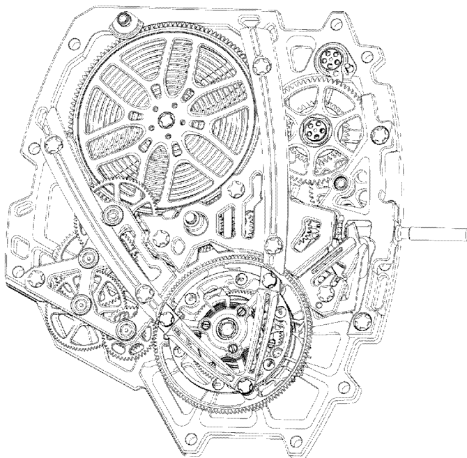
【立體圖1】
