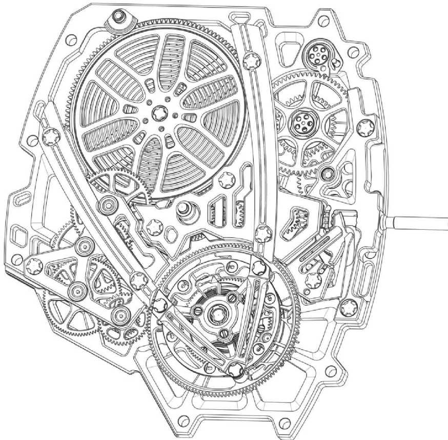
【立體圖1】
