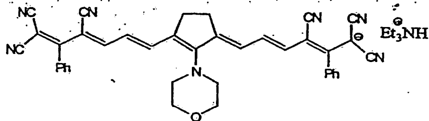
IR-Farbstoff 14
