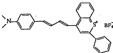
IR-Farbstoff 5
