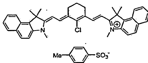
Colorant IR 1
