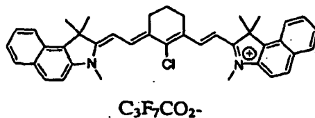
IR Dye 2
