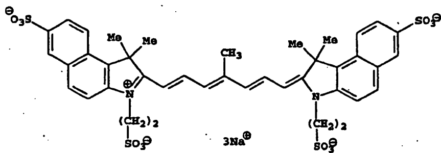
IR Dye 10
