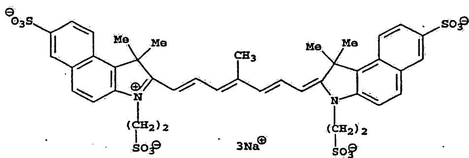
IR-Farbstoff 10
