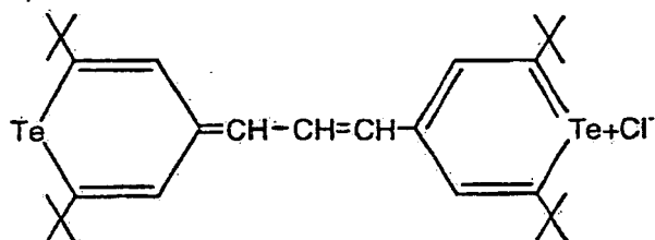
IR-Farbstoff 3
