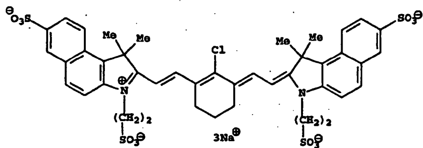
IR Dye 9
