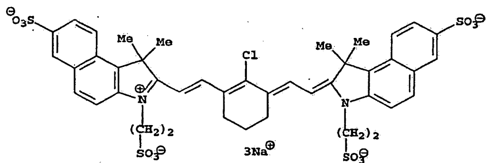
IR-Farbstoff 9
