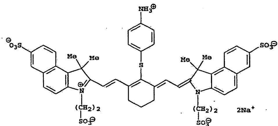
IR-Farbstoff 12
