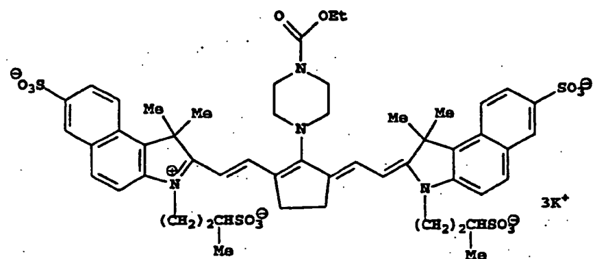
IR Dye 13
