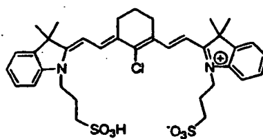
IR Dye 6
