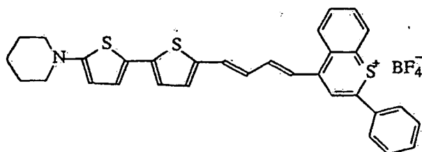
IR-Farbstoff 4
