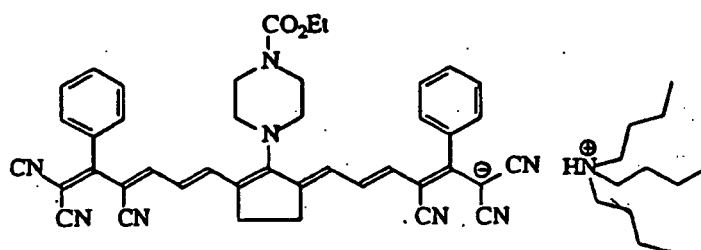
IR Dye 7
