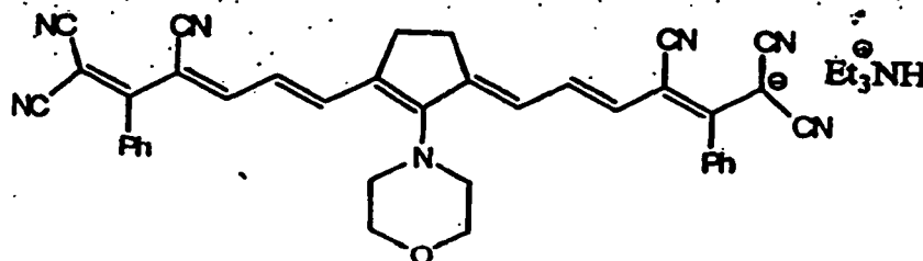
IR Dye 14
