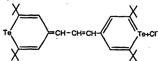
IR Dye 3
