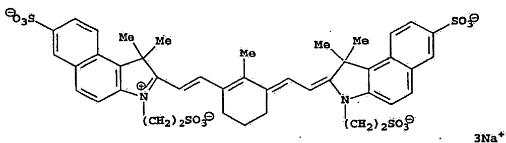
IR-Farbstoff 8
