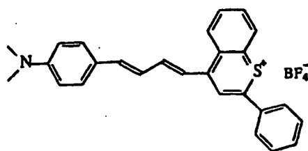
IR Dye 5
