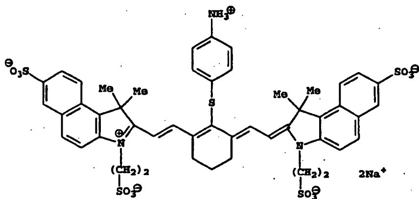
IR Dye 12
