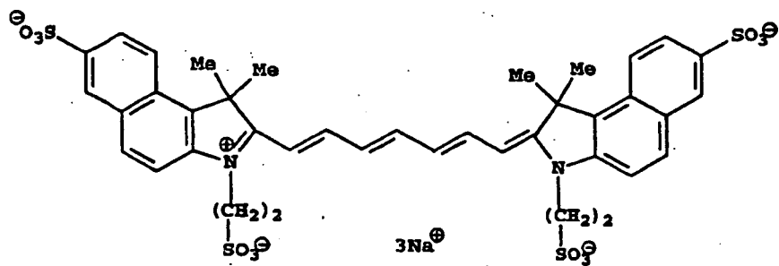
IR Dye 11
