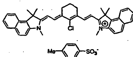
IR Dye 1
