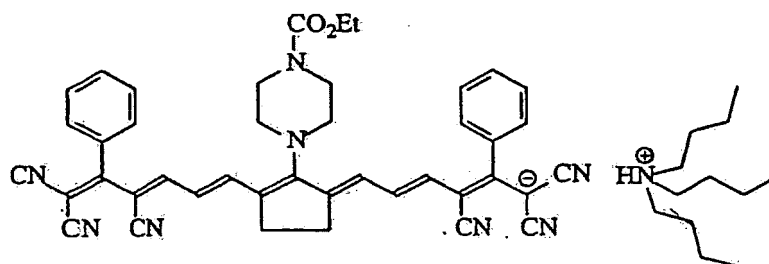
IR-Farbstoff 7
