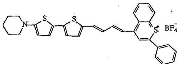
Colorant IR 4
