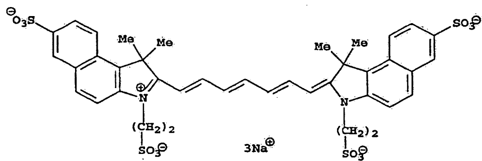
IR-Farbstoff 11
