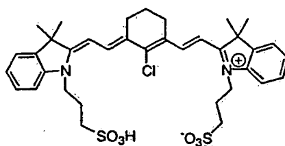
Colorant IR 5
