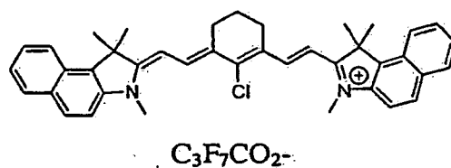
Colorant IR 1
