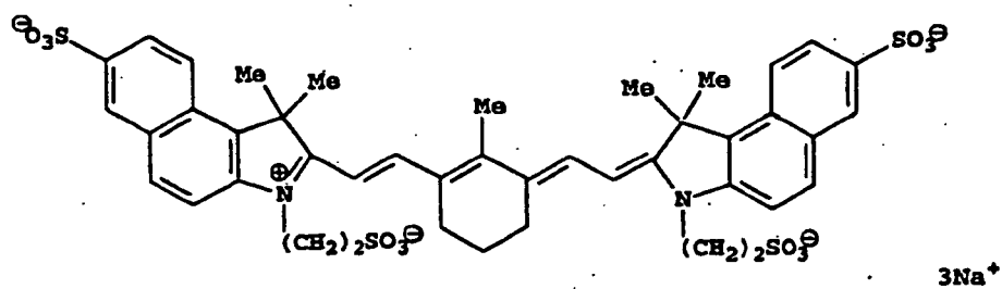
IR Dye 8
