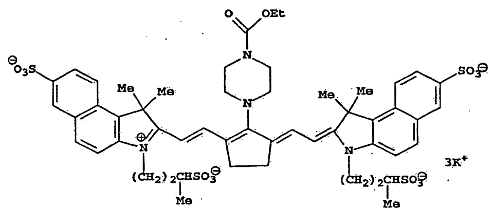
IR-Farbstoff 13
