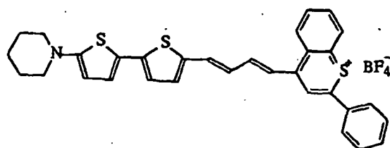
IR Dye 4
