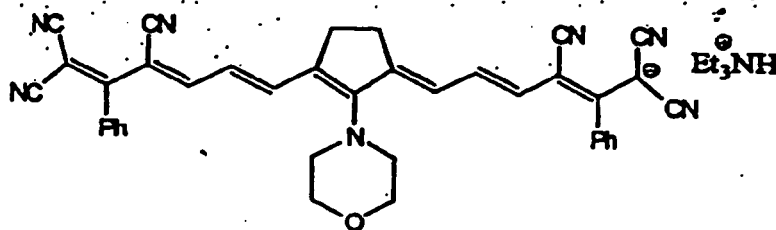
IR Dye 14
