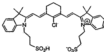
IR-Farbstoff 6
