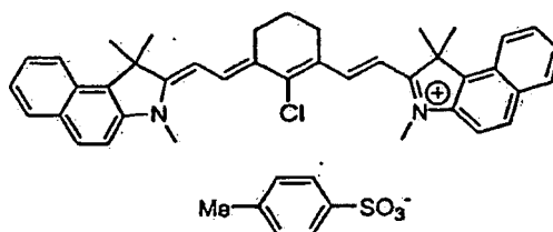
IR-Farbstoff 1
