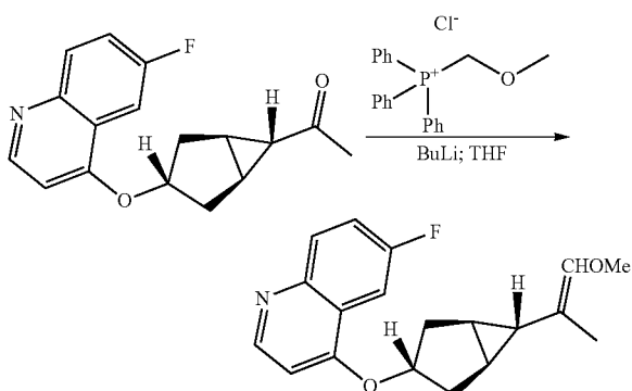
6-Fluoro-4-(((1R,3s,5S,6r)-6-((E)-1-methoxyprop-1-en-2-yl)bicyclo[3.1.0]hexan-3-yl)oxy)quinoline
