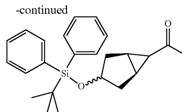
1-((1R,5S)-3-((tert-butyl)phenyl)silyloxy)bicyclo[3.1.0]hexan-6-yl)ethan-1-one
