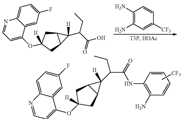
N-(2-amino-4-(trifluoromethyl)phenyl)-2-(((1R,3s,5S,6r)-3-((6-fluoroquinolin-4-yl)oxy)bicyclo[3.1.0]hexan-6-yl)butanamide
