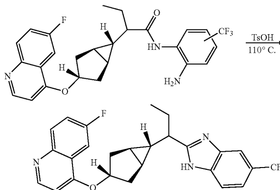
6-Fluoro-4-(((1R,3s,5S,6r)-6-(1-(6-(trifluoromethyl)-1H-benzo[d]imidazol-2-yl)-propyl)bicyclo[3.1.0]hexan-3-yl)oxy)quinoline
