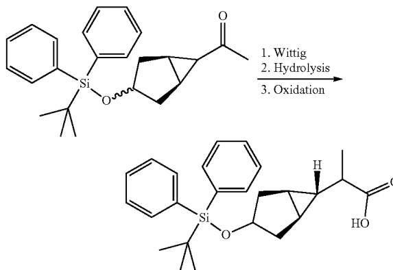
2-((1R,5S,6r)-3-((tert-butyl)phenyl)silyloxy)bicyclo[3.1.0]hexan-6-yl)propanoic acid
