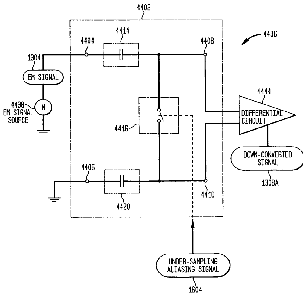
FIG. 44E EXAMPLE INPUT/OUTPUT CIRCUITRY
