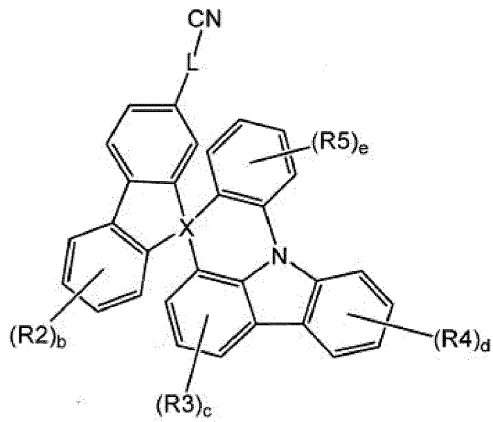
[Formule chimique 1-1]
