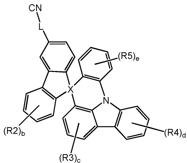
[Chemische Formel 1-2]
