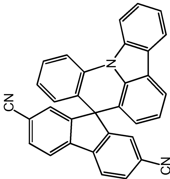
Chemische Formel 2-3
