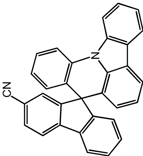
Chemische Formel 2-1
