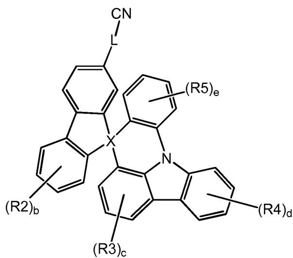
[Chemische Formel 1-2]
