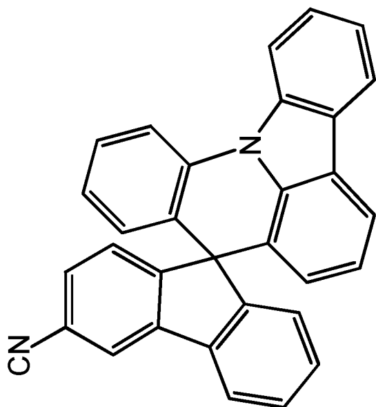
Chemische Formel 2-4
