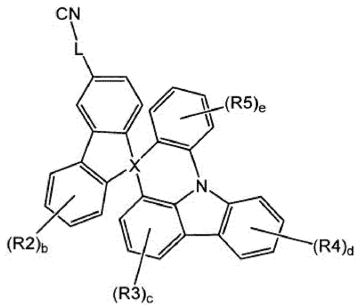
[Formule chimique 1-2]
