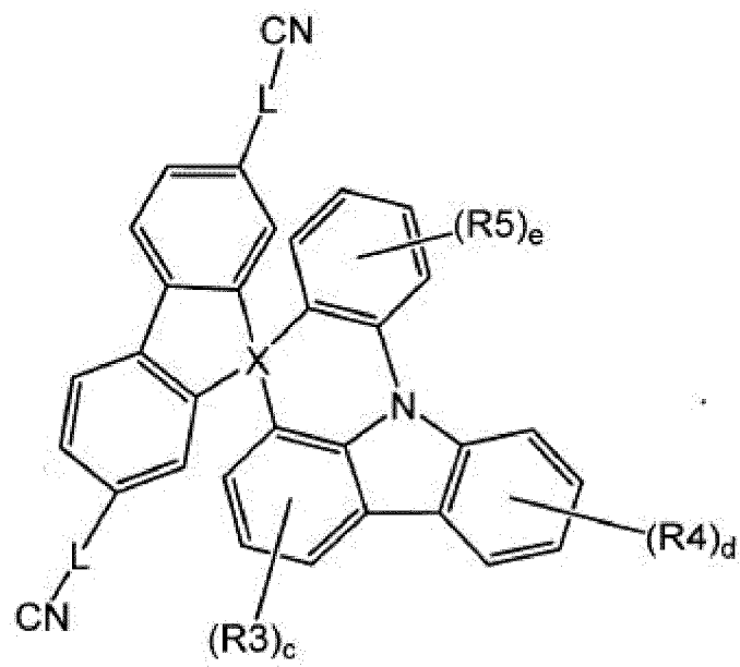
[Formule chimique 1-3]
