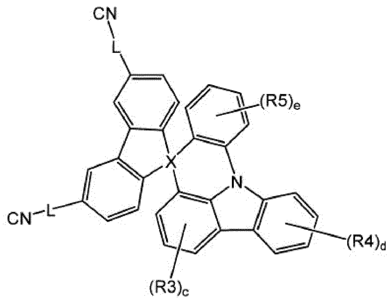
[Formule chimique 1-4]
