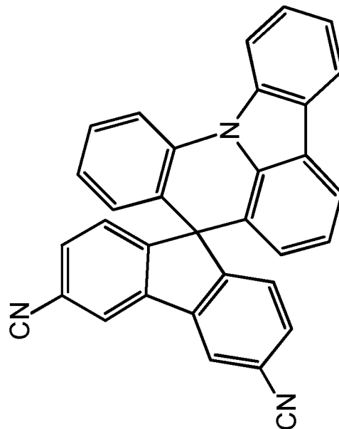
Chemische Formel 2-4
