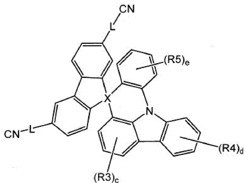
[Formule chimique 1-5]
