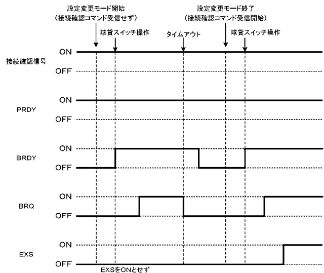
【図9-30】 第4の球貸制限方法
