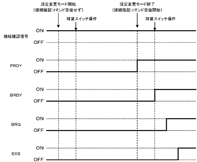
【図9-28】 第2の球貸制限方法
