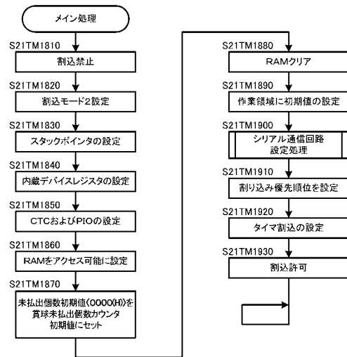
【図9-23】 払出制御メイン処理
