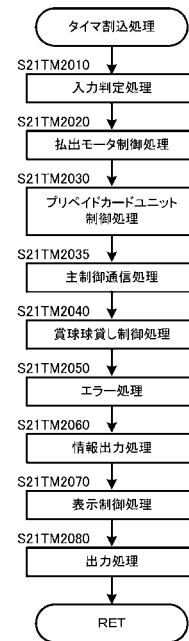
【図9-24】 払出制御タイマ割込処理
