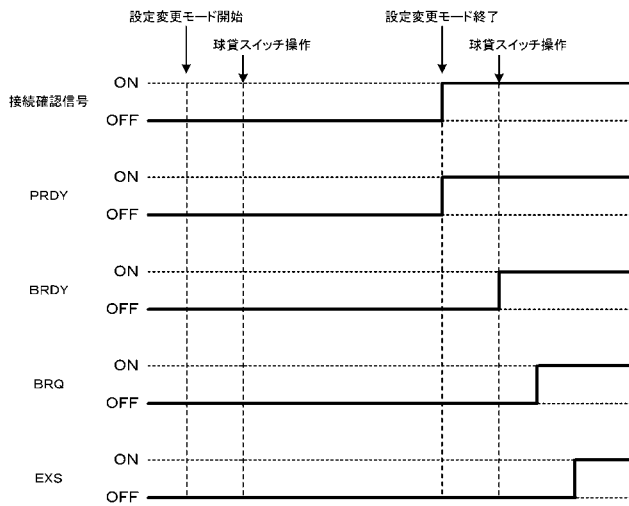
【図9-27】 第1の球貸制限方法
