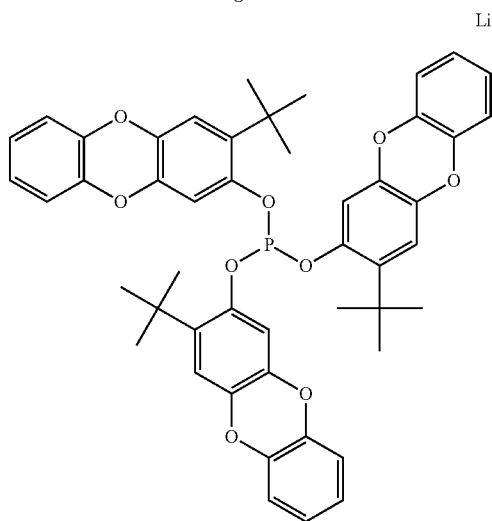
Ligand J
