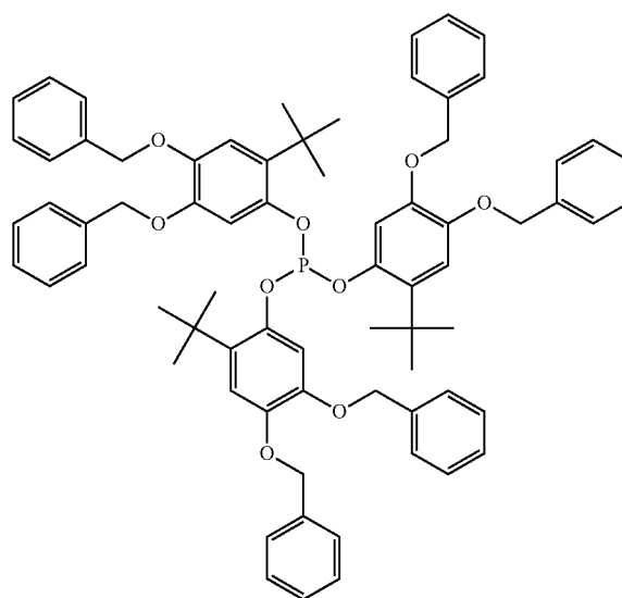
Ligand F
