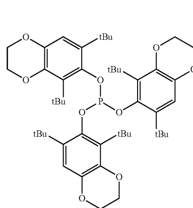
Ligand G
