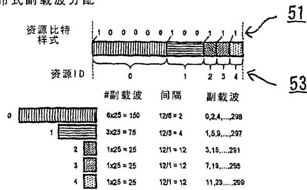
分布式副载波分配
