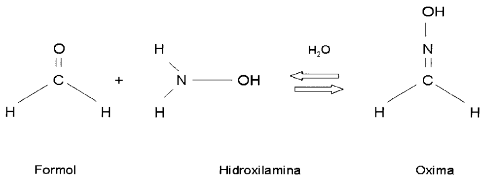
Figura 3. Reacción formaldehído - sulfato de hidroxilamina.
