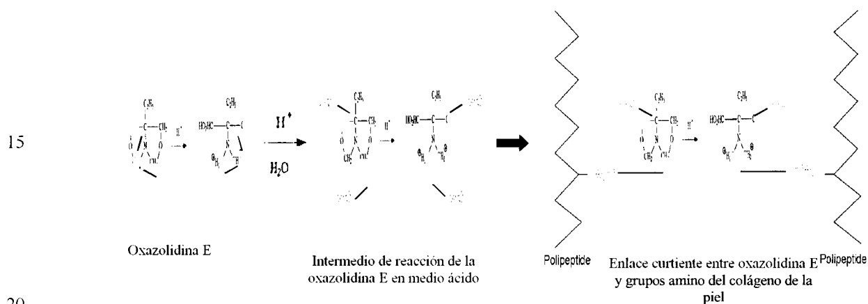
Figura 1. Enlace curtiante colágeno oxazolidina.
