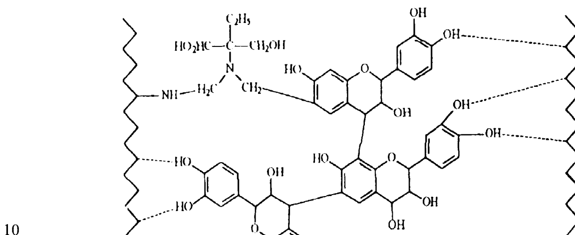
Figura 2. Enlace curtiente colágeno – oxazolidina – curtiente sintético / vegetal.
