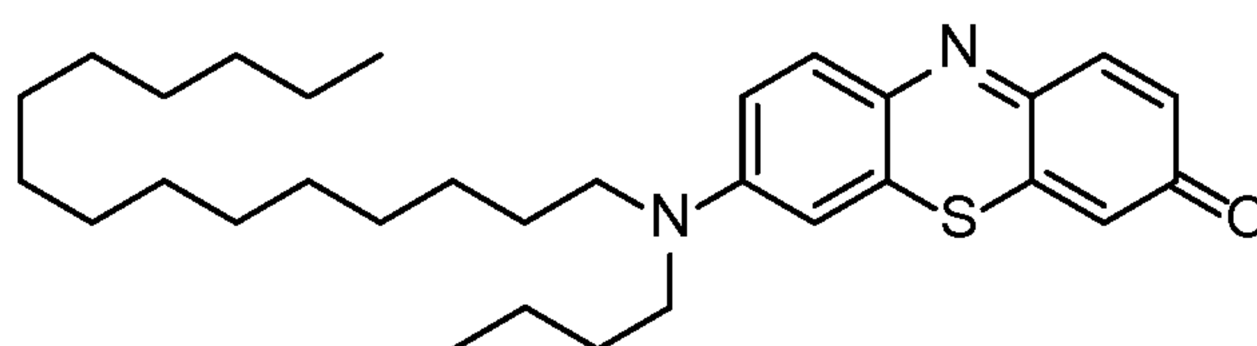
7-(butyl(pentadecyl)amino)-3H-phenothiazin-3-one (33)
