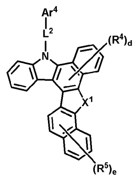
(화학식 37)
