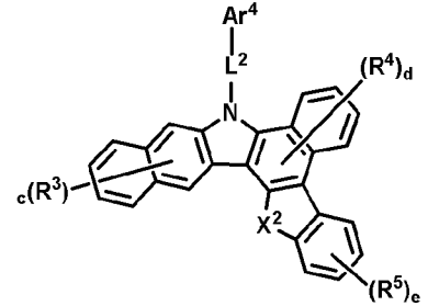
(화학식 43)
