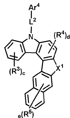
(화학식 34)
