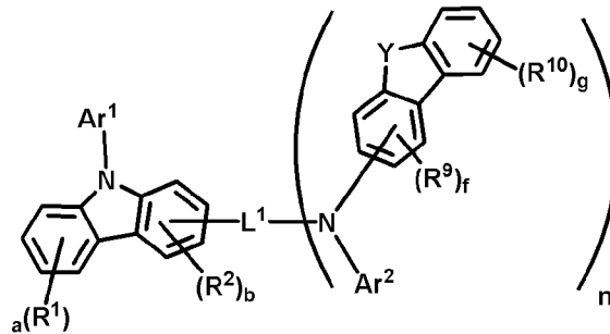
(화학식 23)
