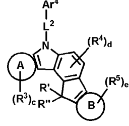
(화학식 52)
