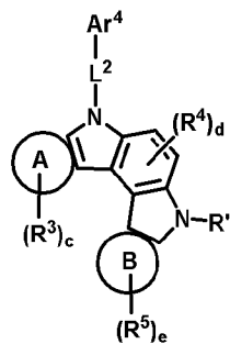
(화학식 46)
