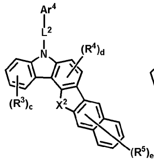
(화학식 44)
