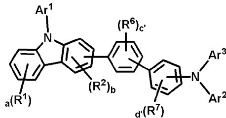
(화학식 7)
