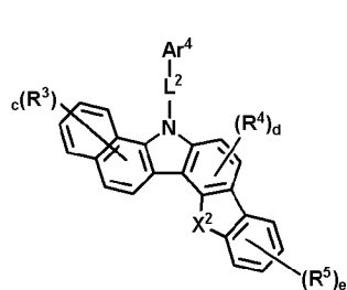
(화학식 36)
