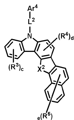
(화학식 40)
