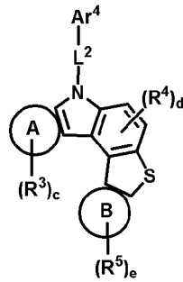
(화학식 47)
