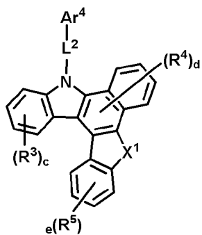
(화학식 29)
