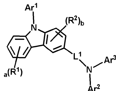
(화학식 4)
