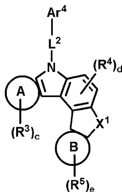
(화학식 24)
