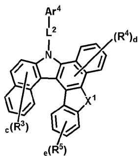
(화학식 36)
