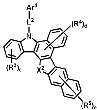
(화학식 44)
