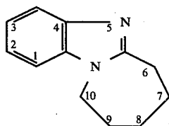
7,8,9,10-tetrahydro- 6H-azepino(1,2-a) benzimidazole
