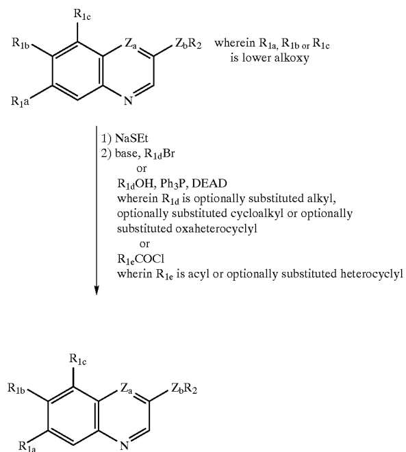
Scheme VI
