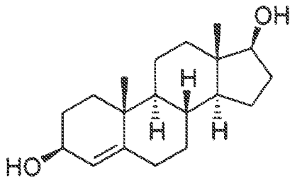
4-Androstenediol
