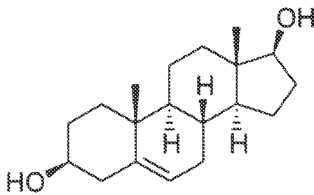
5-Androstenediol
