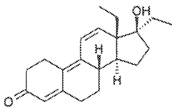
Tetrahydrogestrinone
