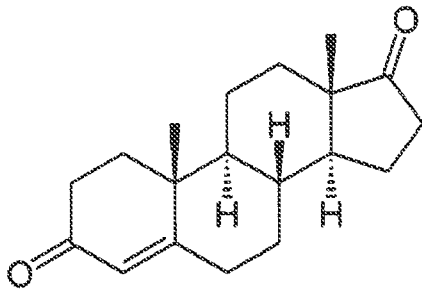
Androstenedione
