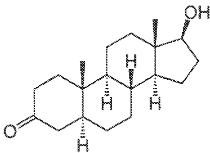
DHT
