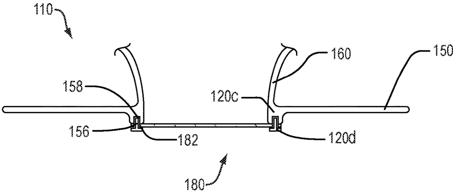
FIG. 5D
