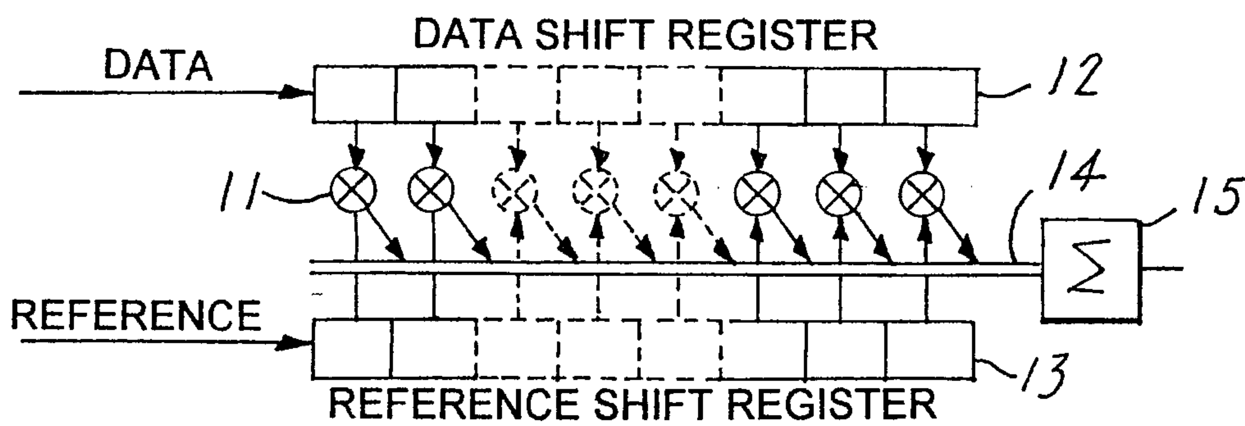
FIG. 2b---PRIOR ART
