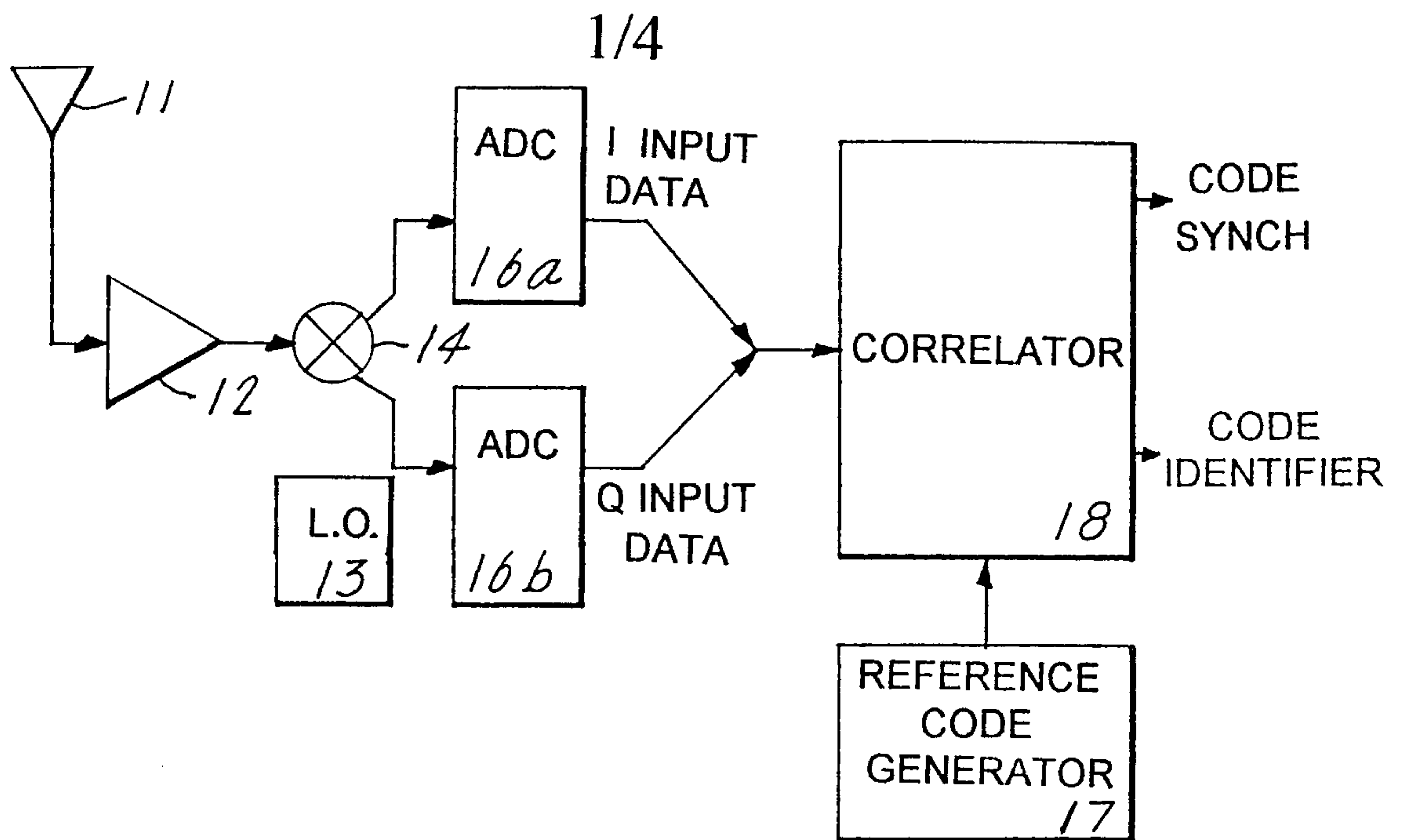
FIG. 1---PRIOR ART
