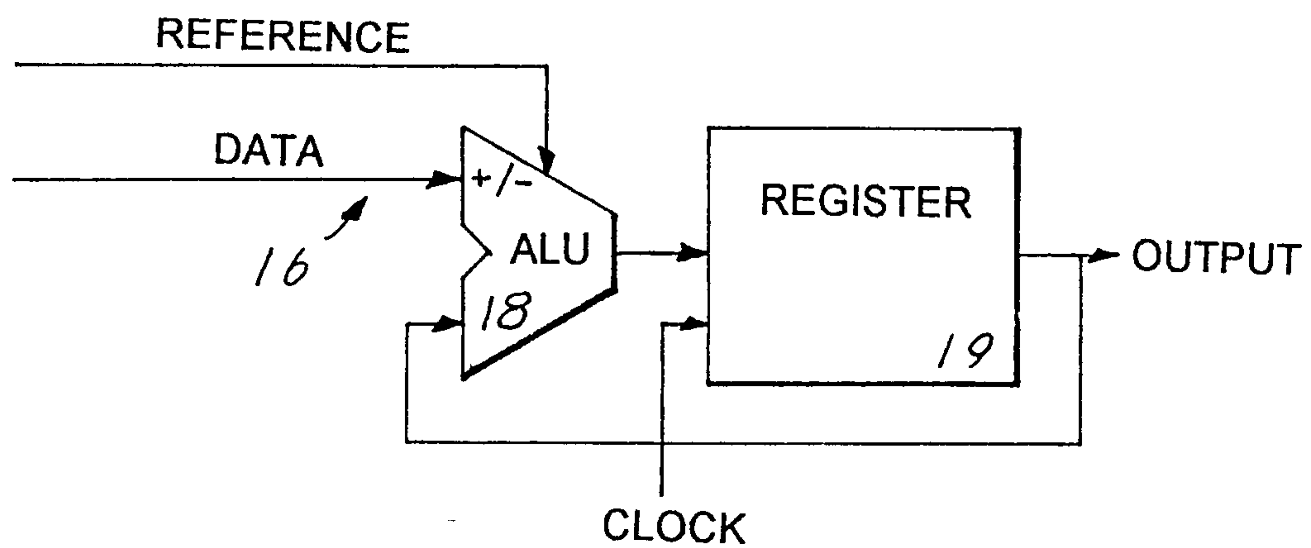
FIG. 2a---PRIOR ART
