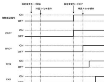
【図10-27】 第1の球貸制御方法
