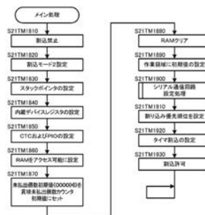
【図10-23】払出制御メイン処理
