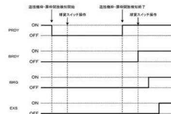
【図10-29】 第3の球貸制御方法
