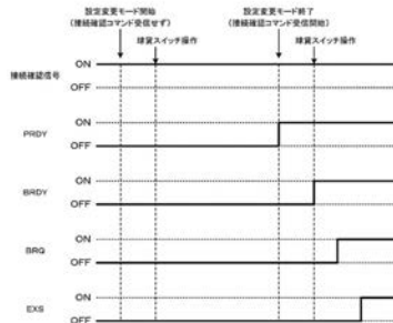
【図10-28】 第2の球貸制御方法
