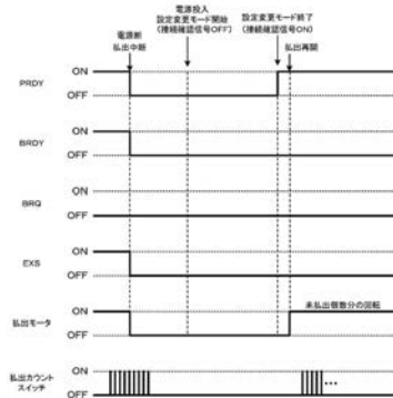
【図10-32】 設定変更モード終了後に球貸を再開
