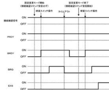
【図10-30】 第4の球貸制御方法
