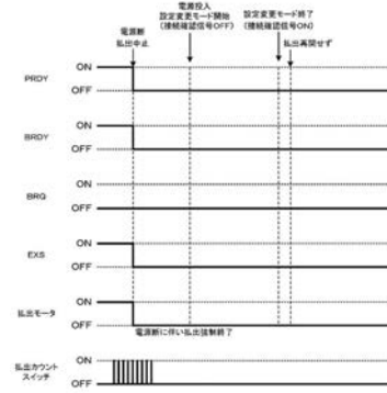
【図10-33】 電源断に伴い球貸を強制終了
