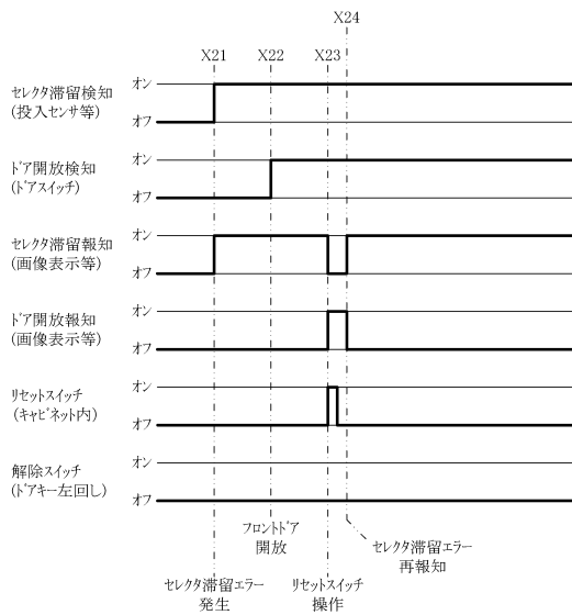
<第9実施形態> エラーの検知時及び解除時の動作態様を示すタイムチャート(2) セレクト滞留エラーの要因を除去せずにリセットスイッチを操作したときの動作態様
