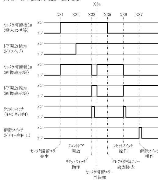
<第9実施形態> エラーの検知時及び解除時の動作態様を示すタイムチャート(3) セレクト滞留エラーの要因を除去せずにリセットスイッチを操作したとき、セレクト滞留エラーの要因除去後にリセットスイッチを操作したとき、及びフロントドアを開放したまま解除スイッチを操作したときの動作態様
