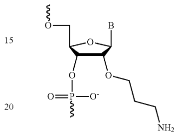
2'-AP
