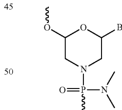
Morpholino
