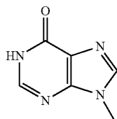
Inosine
