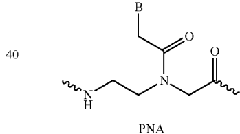
PNA
