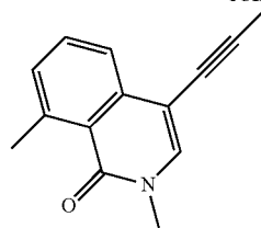
PIM
