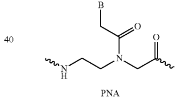
PNA
