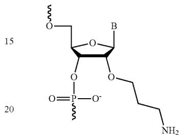
2'-AP
