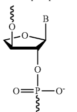
TNA
