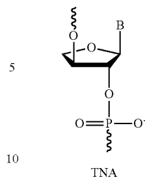
TNA
