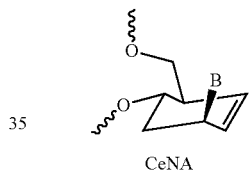
CeNA
