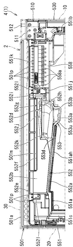
B1-B1断面図
