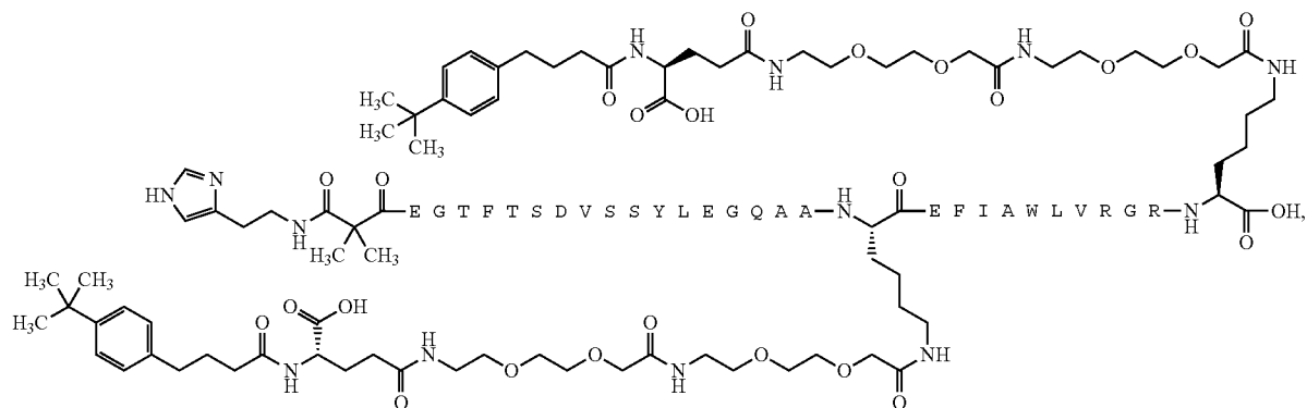
Chem. 46:
