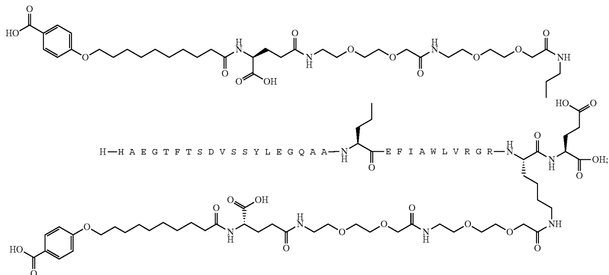
Chem. 64:
