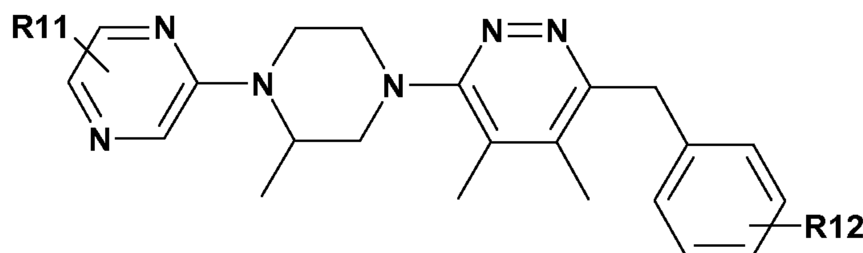
(Ia)
