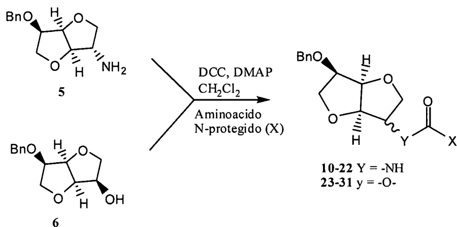
Esquema 4. Síntese dos compostos ( 10-22 ) e ( 23-31 )
