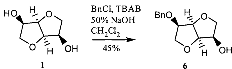
Esquema 3. Síntese do derivado mono benzilado ( 6 ).
