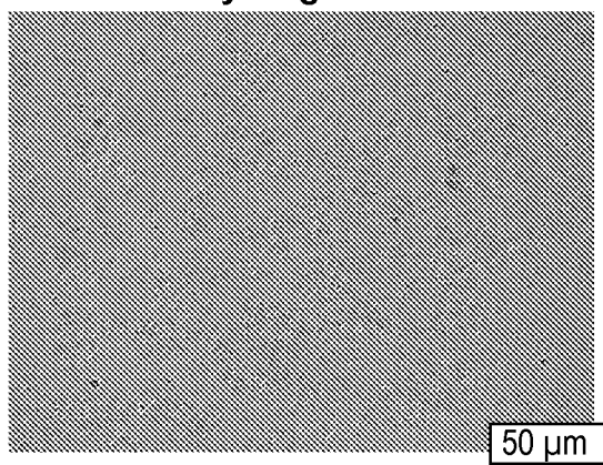
B. OVA/Alhydrogel™
