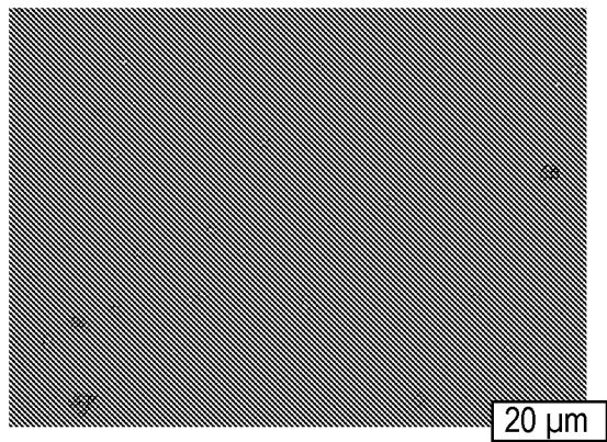
A. OVA/AlPO 4
