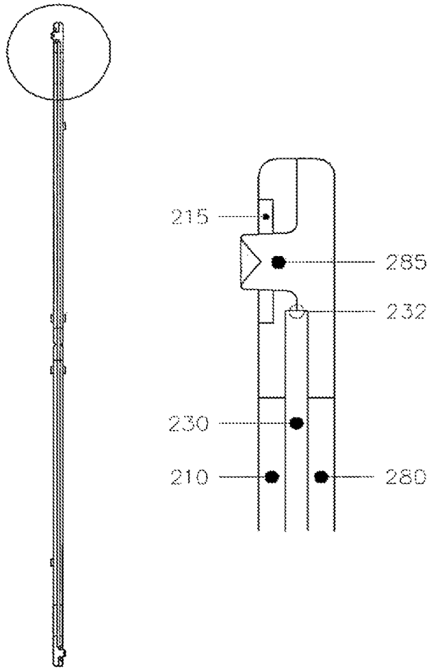
Section A-A
