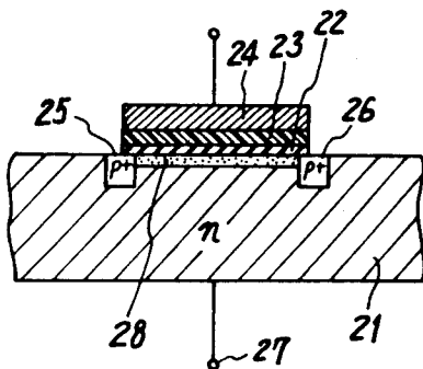
FIG. 1 (p-channel MNOS FET)
