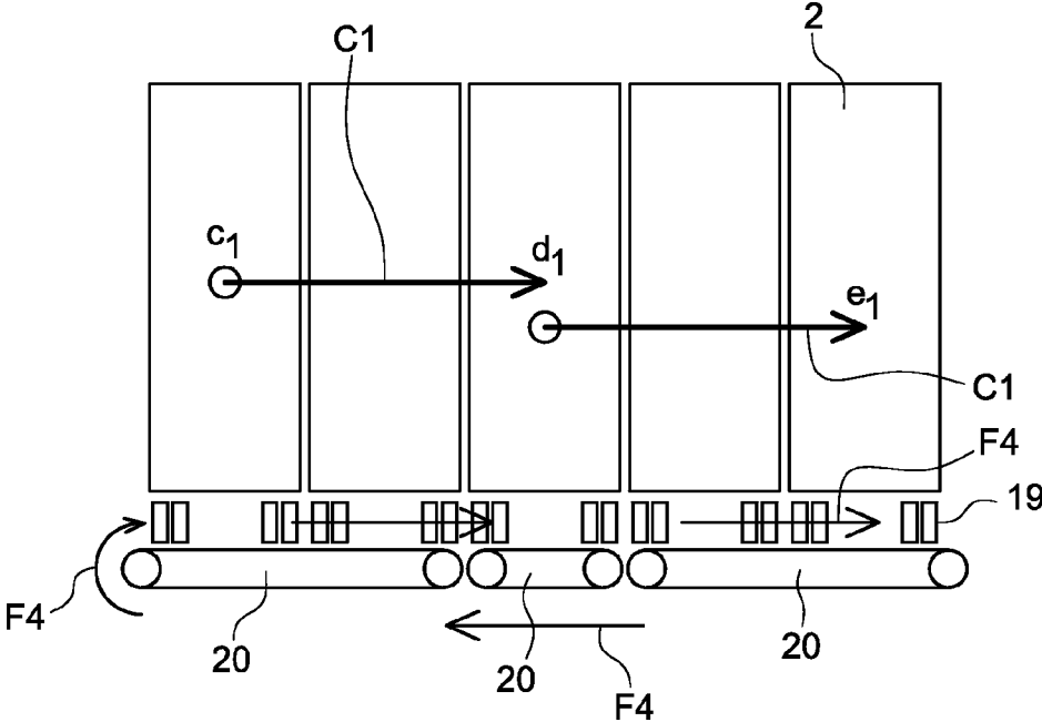
FIG. 10D
